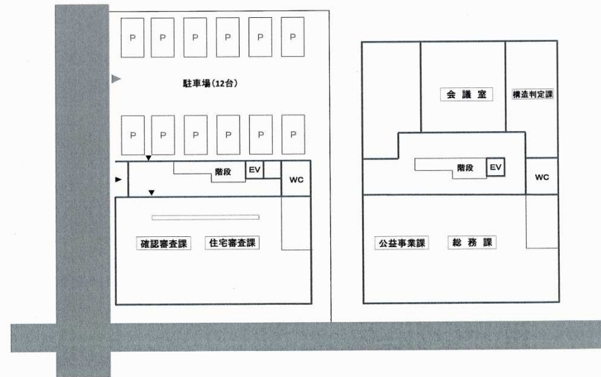
1階見取図
